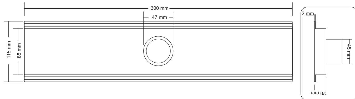
VISTA FRONTAL SAÍDA CENTRAL
