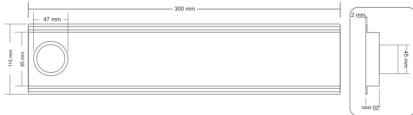
VISTA SUPERIOR CALHA SAÍDA PADRÃO
