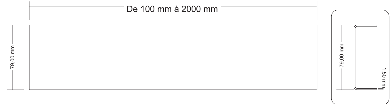
VISTA SUPERIOR TAMPA INOX OCULTO
