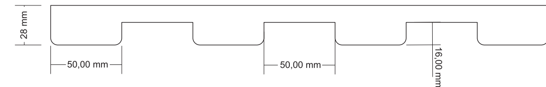
VISTA LATERAL TAMPA INOX OCULTO
